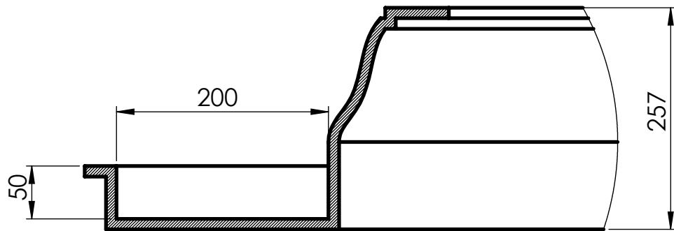
DÉTAIL B ECHELLE 1 : 5
