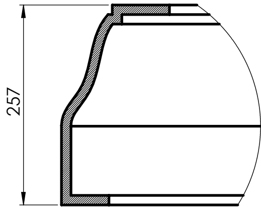
DÉTAIL B Echelle 1 : 4
